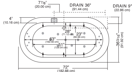
Système Tourbillon et Mass-air / Whirlpool & Mass-air System
